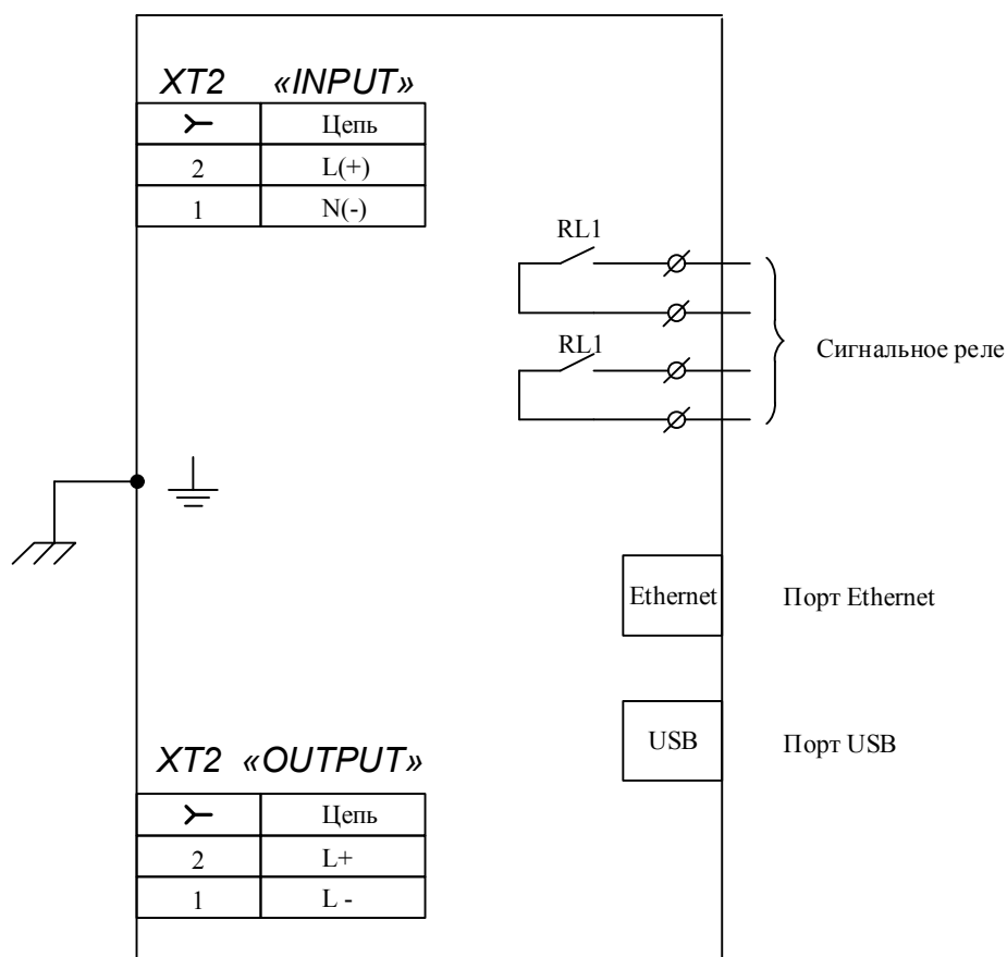
Рисунок 2. Схема внешних подключений
