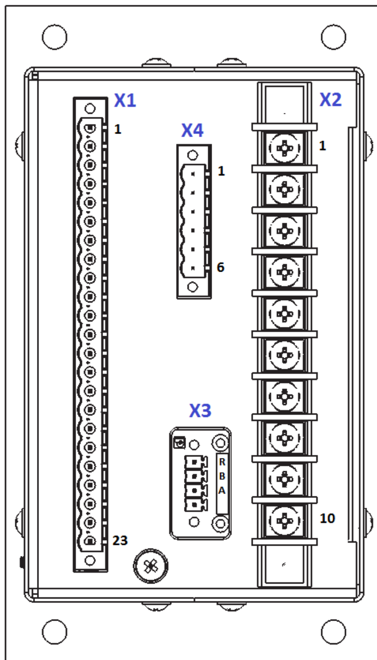
Расположение клеммных зажимов (вид сзади).
