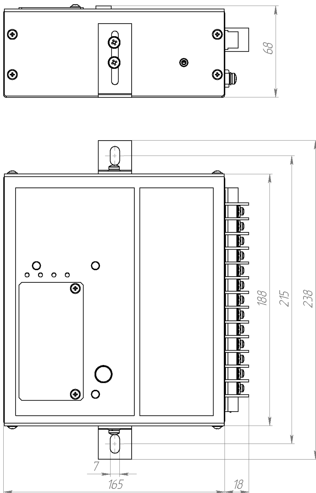
Габаритные и установочные размеры блока REST.01-200, REST.01-200i.
