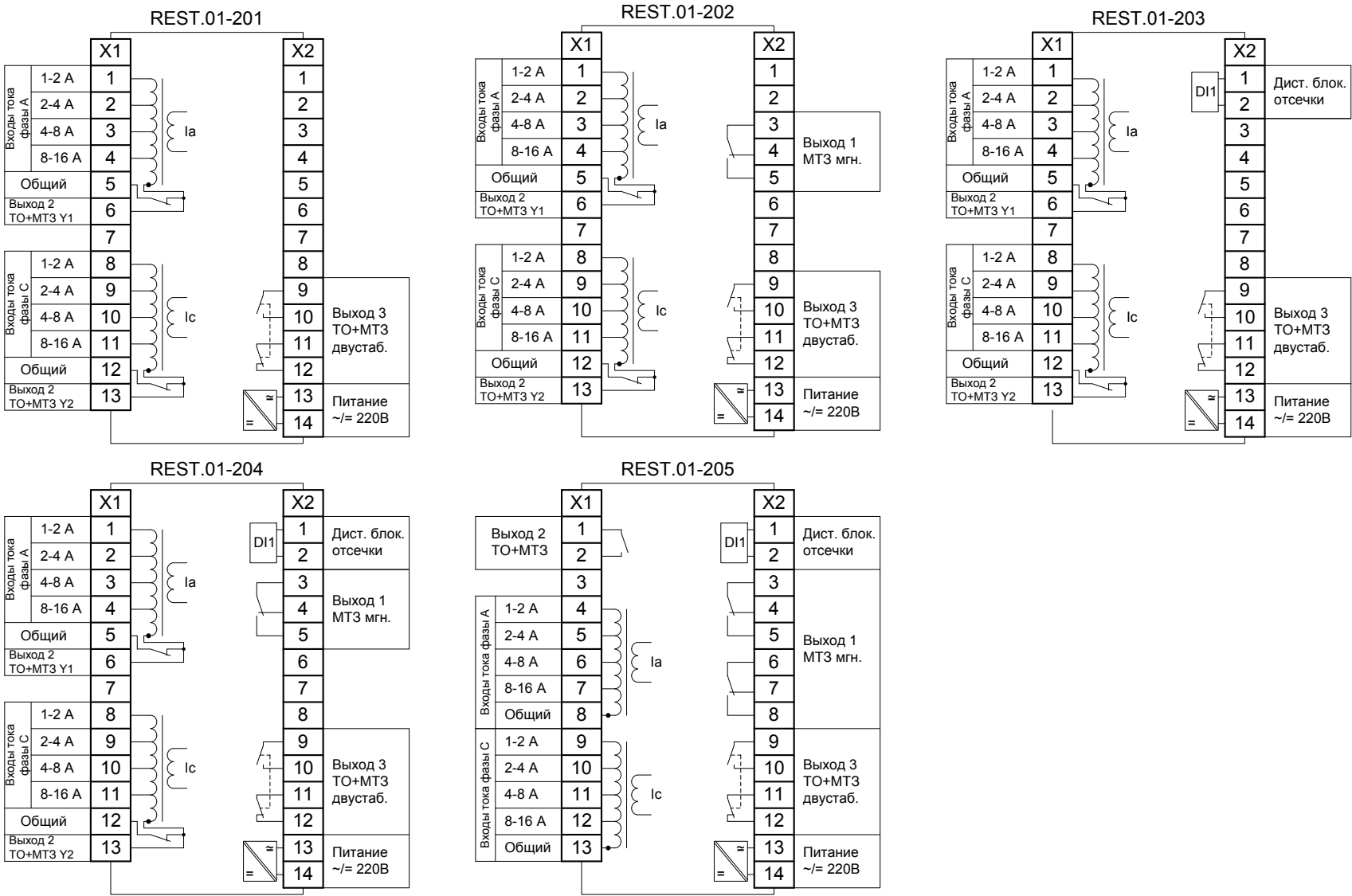
Схемы подключения блоков REST.01-200, REST.01-200i.
