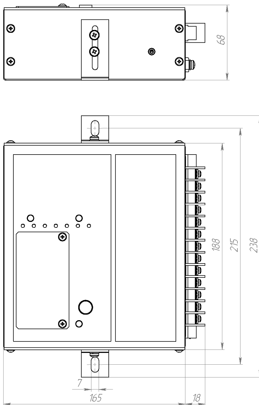
Габаритные и установочные размеры блока REST.01-300.
